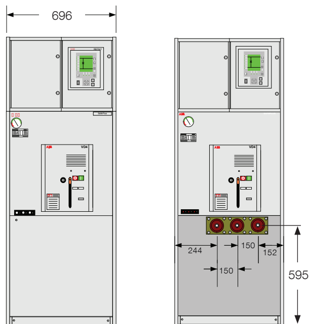
CB modul
